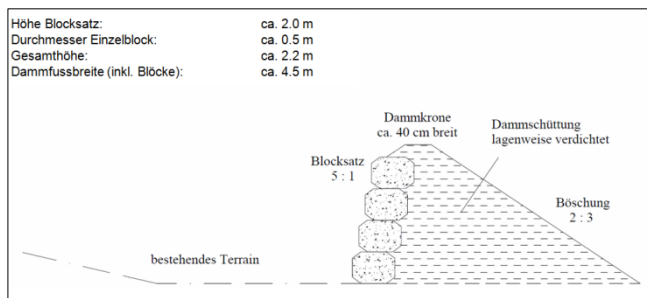
Dimensionierung und Planung: Querschnitt von geplantem Schutzdamm der vor einer Gefährdung durch Sturz- und Hangmuren Ereignisse schützt. Dieser wurde im Rahmen eines Neubaus von einem bestehenden Wohnhaus in Arth geplant.
